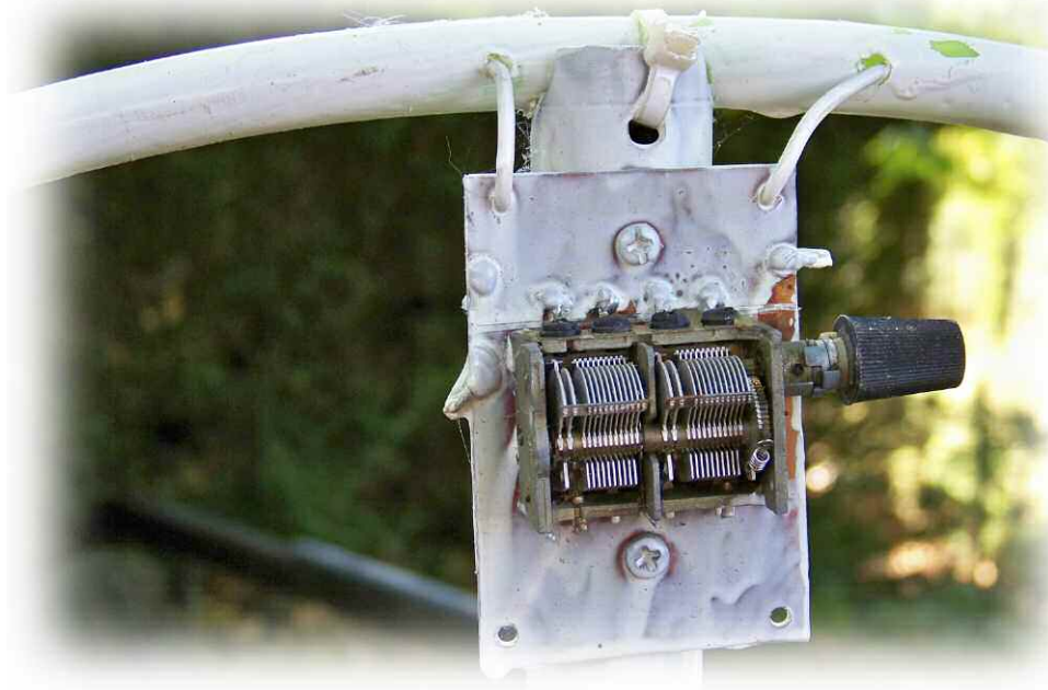
Cette photo montre le gros plan de la partie supérieure de l'antenne boucle, là où se situe le condensateur variable. Attention à l'isolation entre ses lames au cas où vous souhaiteriez pratiquer l'émission avec votre antenne.
